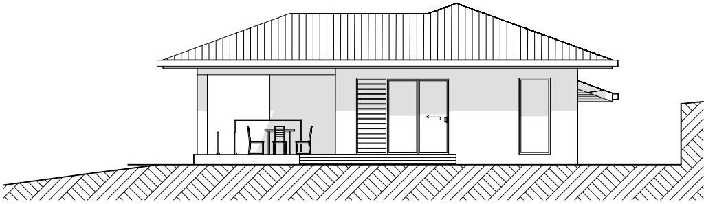
E1 Façade Est 1:150
