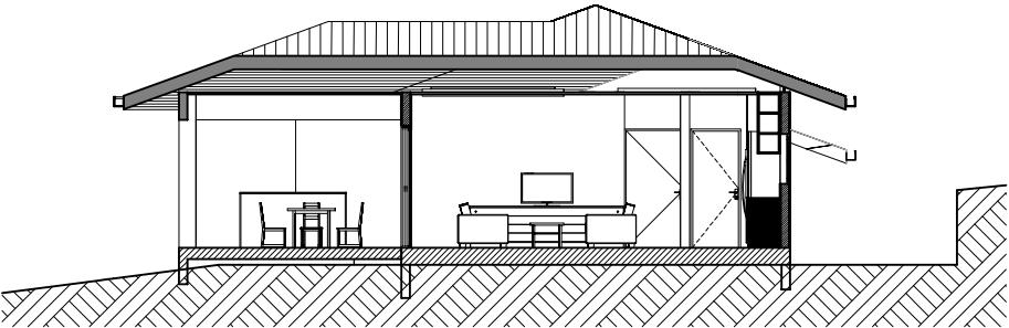
A1 Coupe AA 1:150
