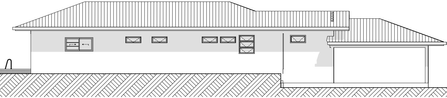
N1 Façade Nord 1:150
